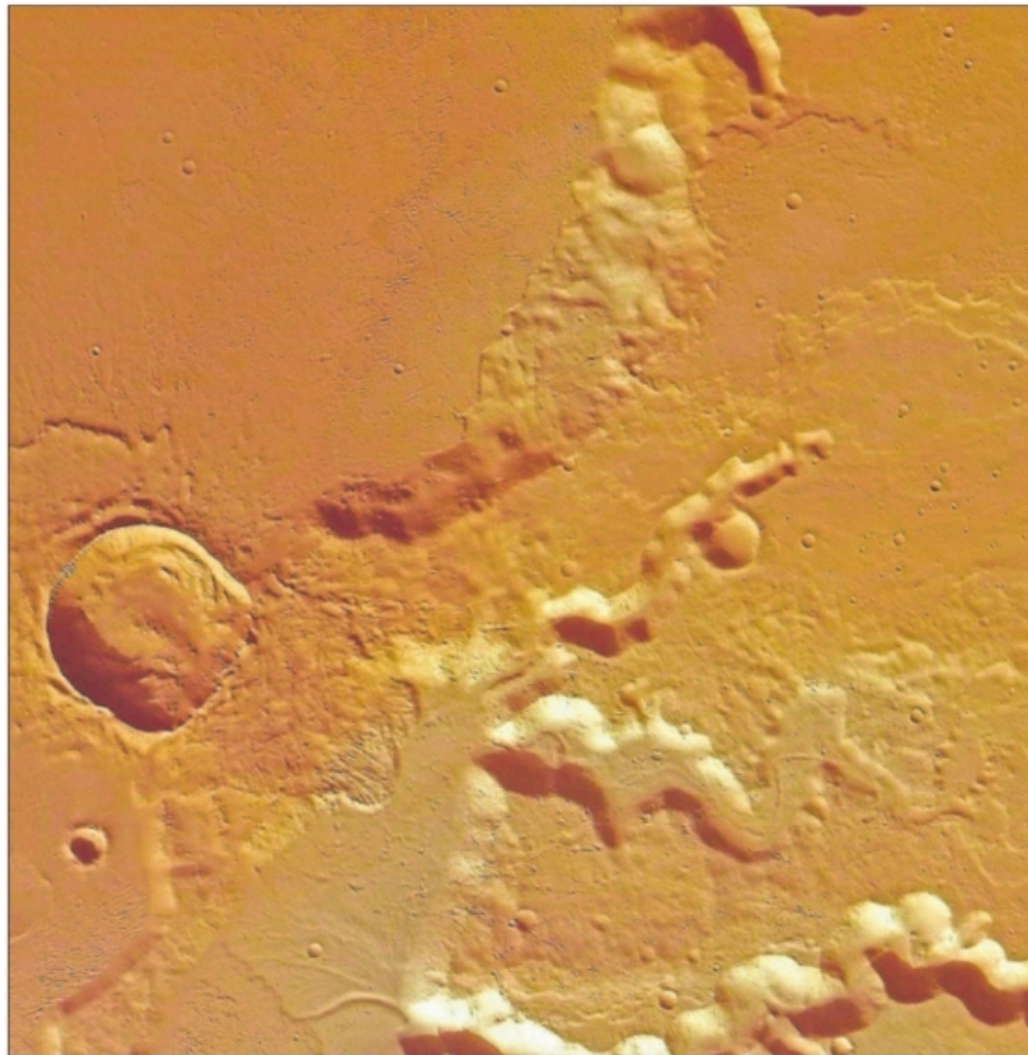
La región Medusa Fossae y áreas adyacentes, en Marte, en una imagen de la Agencia Espacial Europea.
